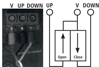
Zaciski przyłączeniowe do zewnętrznych przycisków
