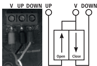
Tilslutningsklemmer til eksterne trykkontakter
