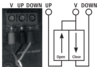
Anslutningsklämmor för extern knapp
