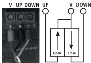
Morsetti di collegamento per i tasti esterni
